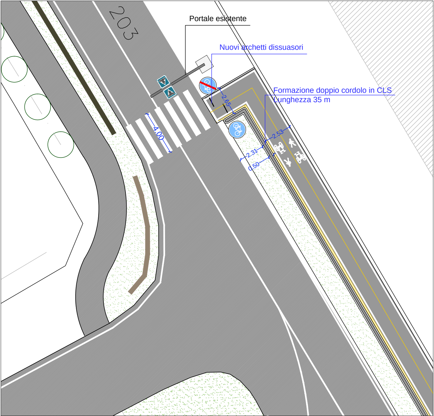
DETTAGLIO PLANIMETRIA DI PROGETTO - scala 1:200
