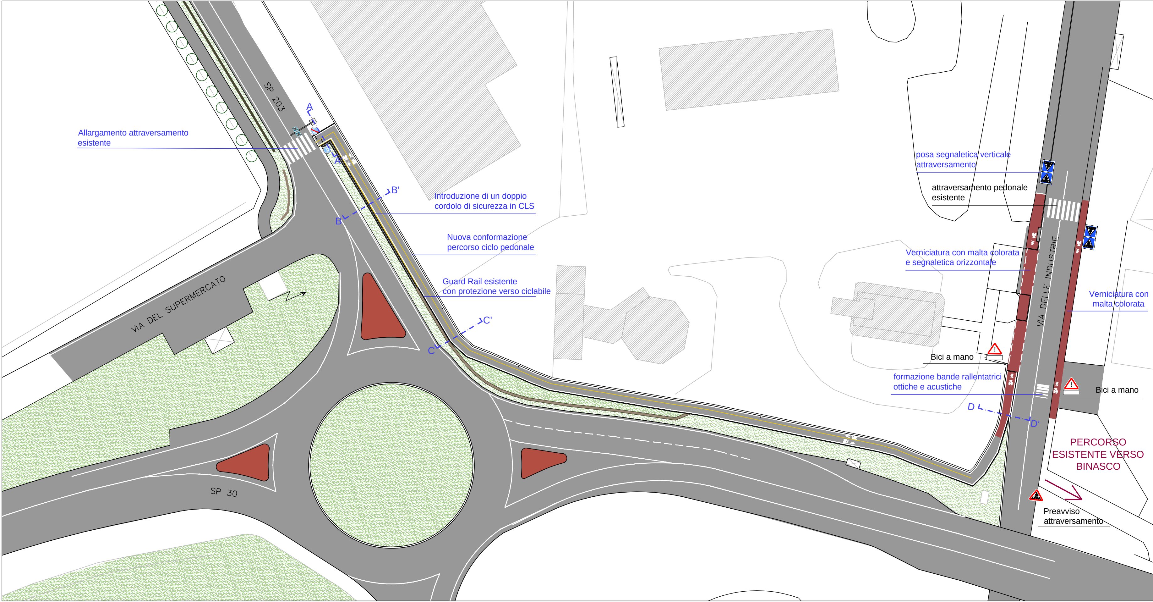
PLANIMETRIA DI PROGETTO - scala 1:500
